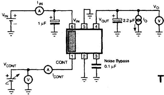
SOT-23L
