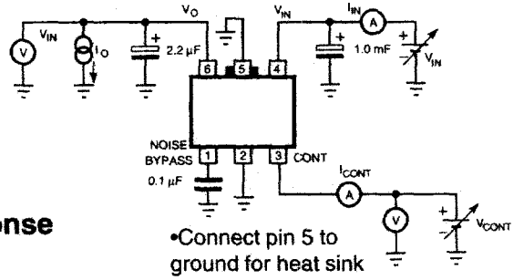
SOT-89-5
